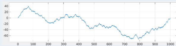
D=2 (d=1, n=1)
